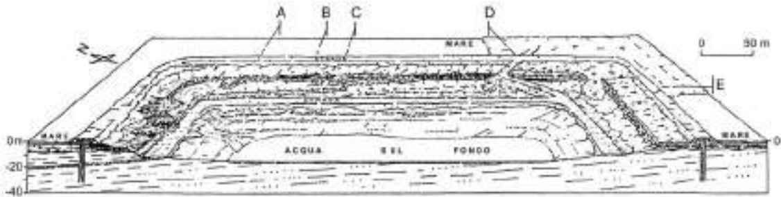
Figura 33 - Stereogramma della metà orientale dello scavo per il Bacino di carenaggio della T. 1 re del Fanale nel Porto di Livorno; le lettere A, B, C, D, E indicano la posizione delle cinque sezioni studiate in particolare (da Barsotti et al., 1974).
