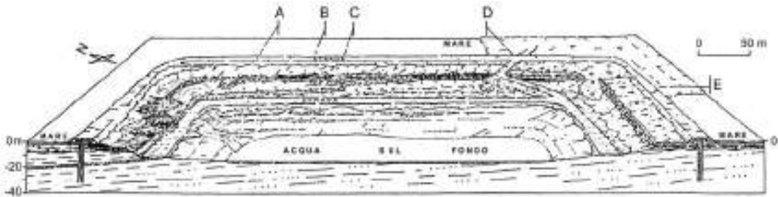
Figura 33 - Stereogramma della metà orientale dello scavo per il Bacino di carenaggio della T. 1ª del Fanale nel Porto di Livorno; le lettere A, B, C, D, E indicano la posizione delle cinque sezioni studiate in particolare (da Barsotti et al., 1974).
