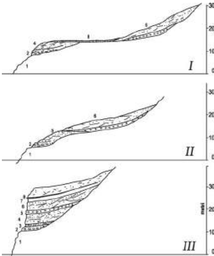
Figura 31 - Tre sezioni nel Pleistocene compreso tra Quercianella e la Buca dei Corvi di Castiglioncello: I - regione più piatta (Quercianella), II - regione intermedia (S. Lucia), III - regione più scoscesa (Buca dei Corvi); 1 - Substrato, 2 - Spiaggia fossile, 3 - Limo rosso, 4 - Duna I, 5 - Breccie, 6 - Duna II, 7 - Loess, 8 - Suolo rosso, 9 - Loess rimaneggiato (da Ottman, 1954). Localizzazione in Figura 30.
