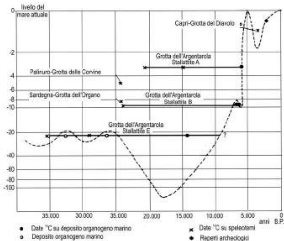
Figura 58 - Curva indicativa delle oscillazioni del livello marino nel Tirreno Centrale per il Pleistocene Superiore-Olocene, le ordinate sono in scala logaritmica (da Alessio et al., 1992).
