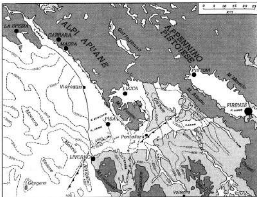
Figura 15 - Isobate del tetto del substrato pre-miocenico rispetto alla superficie topografica: in punteggiato da Ghelardoni et al. (1968), in tratteggiato da Structural Model of Italy (1991) con aggiunte interpretative di faglie sepolte. In grigio scuro gli affioramenti di rocce pre-mioceniche, in grigio chiaro di quelle plioceniche e pleistoceniche, in bianco dei sedimenti alluvionali e delle spiagge (da Della Rocca et al., 1988).
