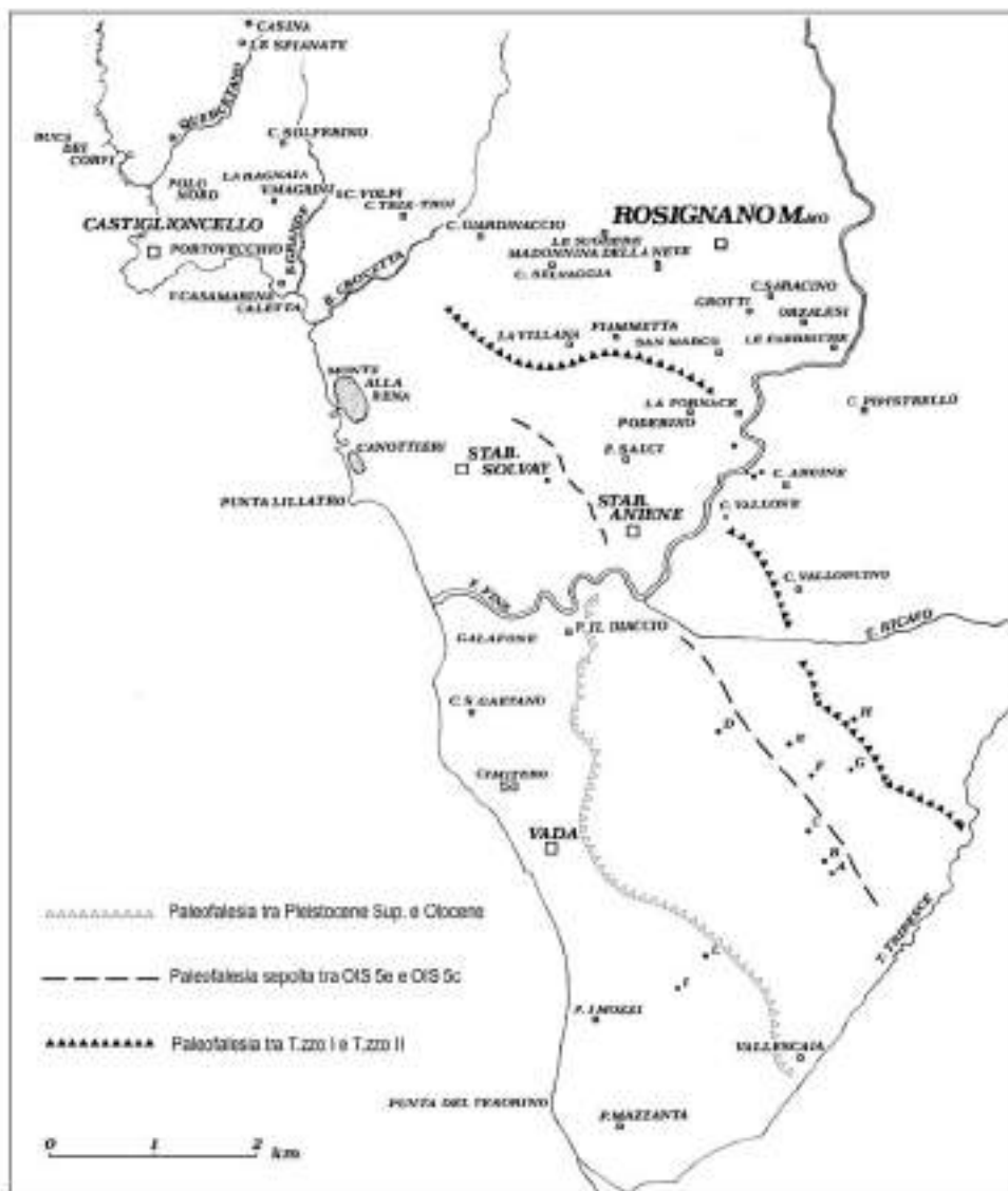
Figura 53 - Ubicazione delle località della parte meridionale del Comune di Rosignano M. mo citate nel testo; le lettere isolate corrispondono alla posizione dei pozzi citati in Figura 54 (da Mazzanti, 2000).
