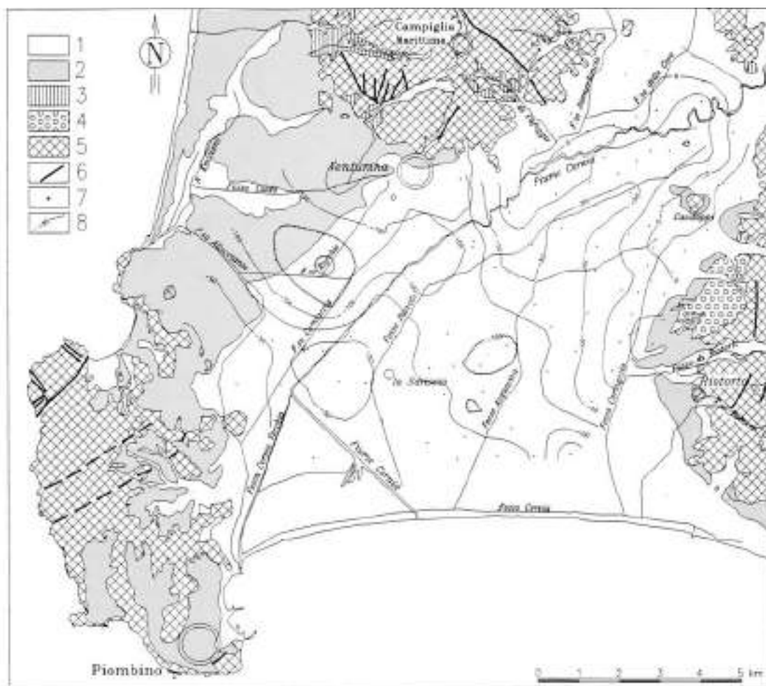
Figura 60 - Carta delle isoipse della superficie sepolta Se_2 . 1 - Sedimenti alluvionali, palustri, lagunari e dei cordoni dunari (Olocene); 2 - Sabbie di Donoratico (Pleistocene Superiore); 3 - Sabbie di Val di Gori, Travertini e Conglomerati di Pod. S. Luigi (Pleistocene Medio); 4 - Conglomerati di Montebamboli (Miocene Superiore); 5 - Insieme delle rocce anteriori al Miocene Superiore; 6 - Faglie; 7 - Indicazione dei sondaggi S.E.V.; 8 - Isoipse della superficie sepolta Se_2 (da Censini et al., 1991).
