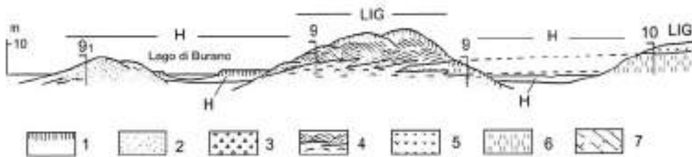
Figura 80 - Sezione stratigrafica attraverso il Lago di Burano; 1 - Suolo, 2 - Duna olocenica (e/o Pleistocene Superiore), 3 Breccia, 4 - Spiaggia alta su duna costiera; 5 - Depositi vulcanici; 6 - Laguna a Cerastoderma ; H - Olocene; L.I.G. - Ultimo interglaciale (da Hearty e Dai Pra, 1986).
