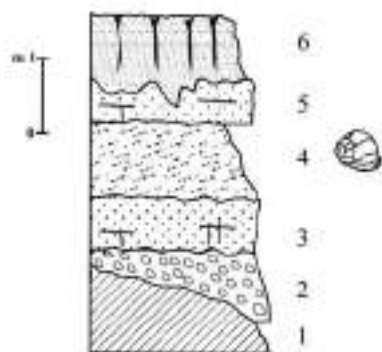
Figura 40 - Sezione stratigrafica di V. la S. Giorgio; 1 – Substrato pre-pleistocenico, 2 – Ghiaie fluviali (Pleistocene Medio ?), 3 – “Panchina I” eolica (OIS 5e), 4 – Sabbie fangose con molluschi non marini, 5 – “Panchina II” eolica (OIS 5c), 6 – Sabbie rosse di Ardenza ormai da considerarsi sinonime delle Sabbie di Donoratico (da Zanchetta et al., 2004).
