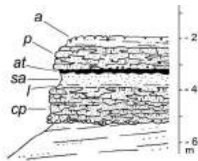
Figura 34 - Particolare della Sezione C di Figura 33, il significato delle lettere è nel testo.
