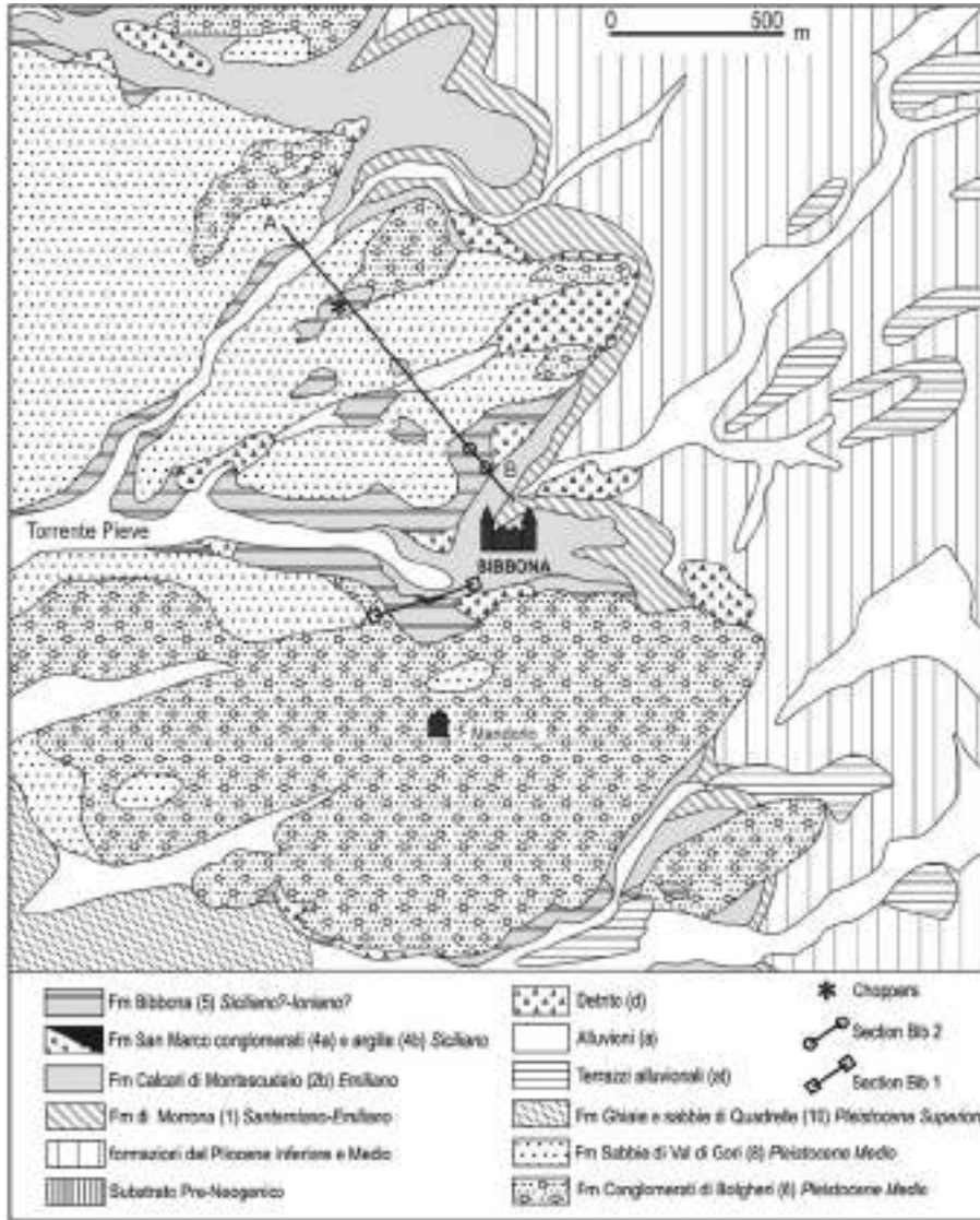
Figura 13 - Carta geologica schematica dei dintorni di Bibbona (da Dall'Antonia et al., 2005).
