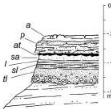
Figura 37 - Particolare della Sezione D di Figura 33, il significato delle lettere è nel testo.
