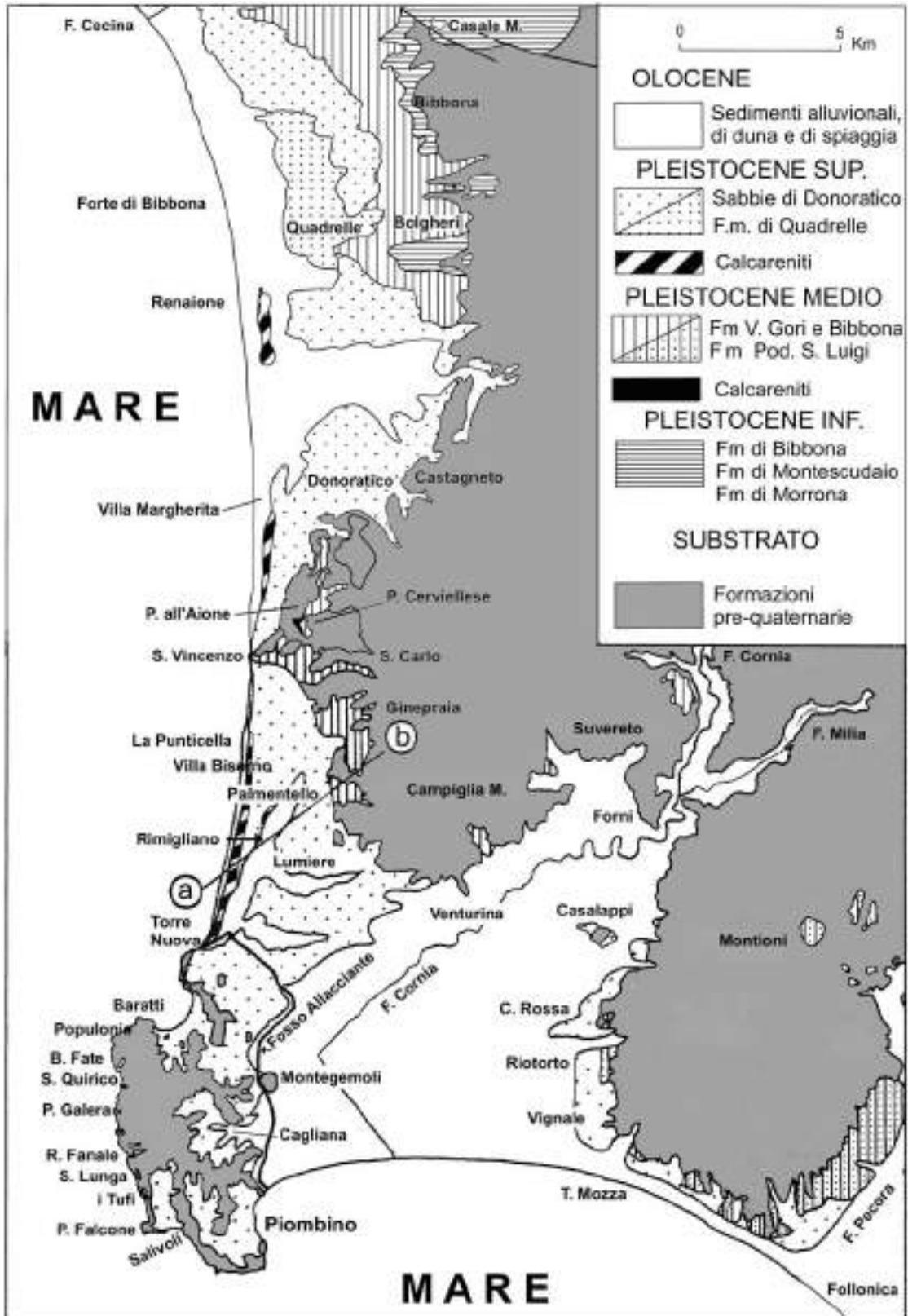
Figura 18 - Carta geologica schematica dell'area compresa tra la Val di Cecina, Piombino e Follonica.
