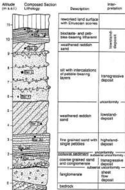
Figura 68 - Colonna stratigrafica ricostruita da Barbara Mauz lungo la falesia della Baia Baratti con la posizione dei campioni raccolti per le determinazioni di età (da Mauz, 1999).
