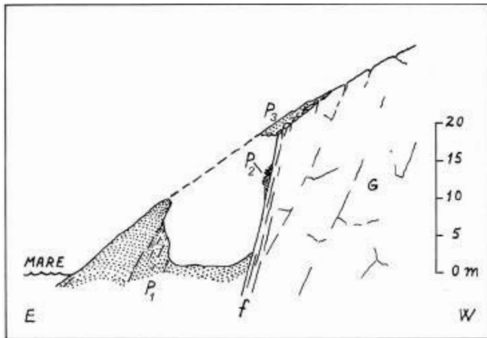
Figura 85 - Isola di Cerboli sezione trasversale a quella di Figura 84 per mostrare che la <Panchina> in P 3 ha sormontato lo specchio della faglia f l'attività della quale va considerata quindi precedente alla deposizione della <Panchina>.
