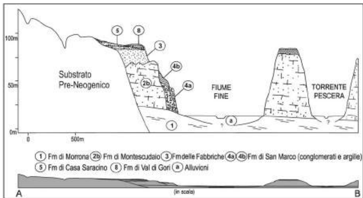
Figura 12 - Sezione geologica A-B di Figura 11 (da Dall'Antonia et al. , 2005).
