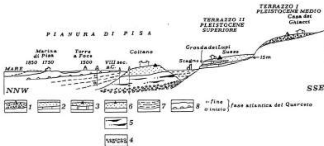
Figura 41 - Sezione geologica (non in scala) fra Marina di Pisa e le C. inc. Livornesi (C. sa dei Ghiacci). 1 - Conglomerati di C. sa P. ino ai Lecci con industrie del Paleolitico Inferiore sul T. ZZO I; 2 - Calcareniti di Castiglioncello e Sabbie di Donoratico sul T. ZZO II; 3 - Calcareniti di Antignano e Sabbie di Donoratico con industria del Paleolitico Medio sul T. ZZO II; 4 - Conglomerati dell'Arno e Serchio da Bientina del Würm I, 5 - Limi e torbe palustri del sottosuolo; 6 - Sabbie di Vicarello con industria del Paleolitico Medio; 7 - Limi e torbe lagunari-palustri e fluviali (Würm III - Olocene almeno nella parte spettante alla Fase Atlantica del Querceto); 8 - Sedimenti litoranei della Trasgressione Versiliana. La linea tratteggiata ad Ovest di Marina di Pisa indica il punto di maggiore sviluppo del litorale raggiunto nel 1850 circa, prima dell'inizio dell'arretramento ancora in atto (da Mazzanti, 1994).
