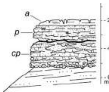
Figura 35 - Particolare della Sezione A di Figura 33, il significato delle lettere è nel testo.
