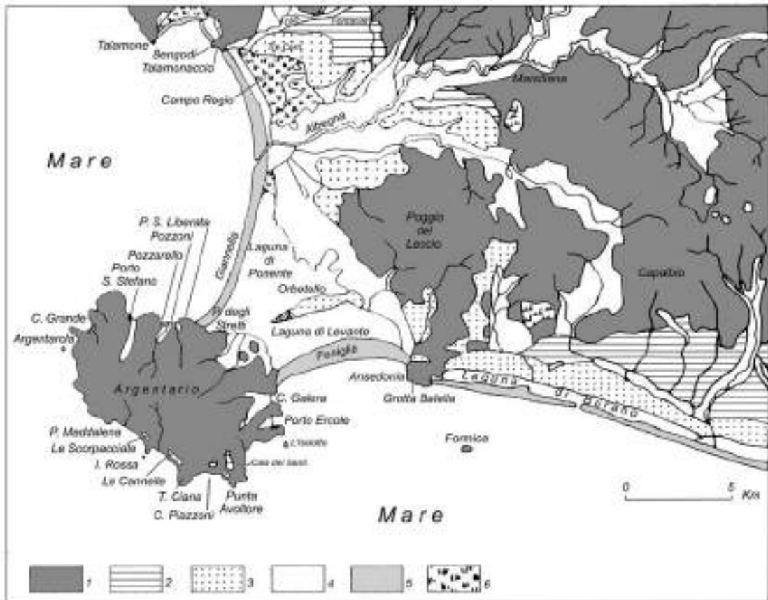
Figura 21 - Carta geologica schematica del tratto meridionale della Toscana Costiera. 1 - Substrato pre-pleistocenico; 2 - Formazioni del Pleistocene Medio; 3 - Formazioni del Pleistocene Superiore. Depositi olocenici: 4 - Sedimenti alluvionali; 5 - Lidi; 6 - Sedimenti palustri.
