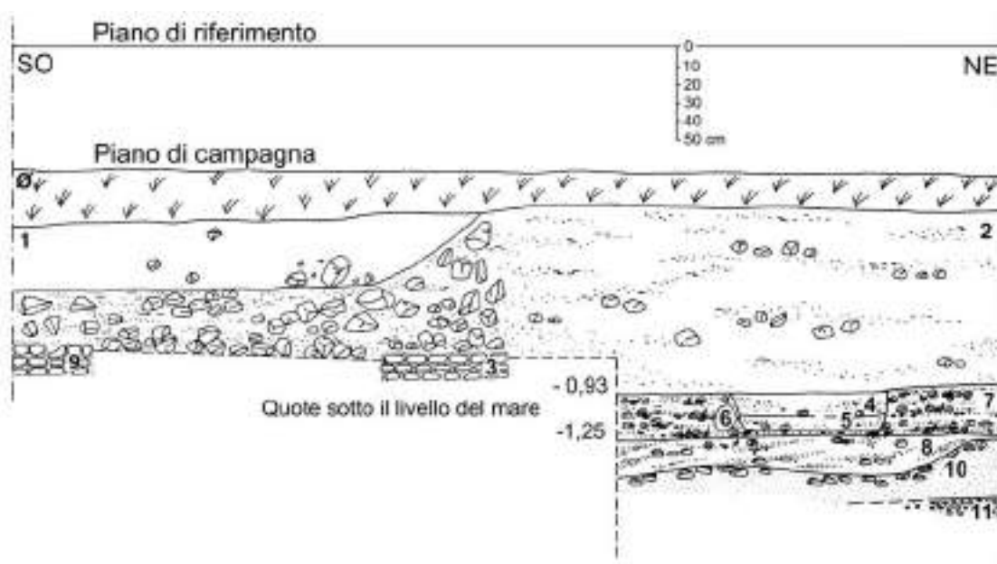
Figura 57 - Sezione lungo il saggio stratigrafico di S. Gaetano di Vada: 0 – terreno agricolo; 1 – strato di manipolazione antropica recente; 2 – sabbia mista a malta disfatta, ciottoli di <Panchina> e materiale eterogeneo anche moderno; 3 – fondazione del muro perimetrale orientale degli horrea ; 4 – sabbia a granuli fini mista a rari piccoli ciottoli appiattiti, di spiaggia, e a scarsi frammenti in ceramica d'impasto; 5 – sedimento analogo al precedente, ancora documentante la frequentazione antropica; 6 – fossa grosso modo circolare; 7 – sabbia con piccoli ciottoli di forma irregolare, mista a numerosissimi fossili di ambiente lagunare a comunicazione con il mare aperto; 8 – sabbia a granuli di dimensioni medie con alcuni fossili (analoghi ai precedenti), lenti arrossate, carboncini e frammenti di ceramica d'impasto; 9 – parte inferiore di un muro divisorio interno degli horrea ; 10 – sabbia a granuli fini misti a numerosissimi frammenti di ceramica d'impasto; 11 – ghiaia a piccoli ciottoli irregolari che corrisponde con il livello della falda freatica (da Mazzanti et al., 1995).
