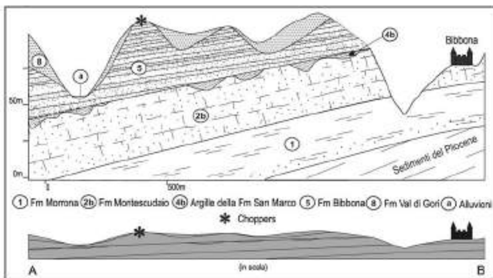
Figura 14 - Sezione geologica A-B di Figura 13 (da Dall'Antonia et al., 2005).
