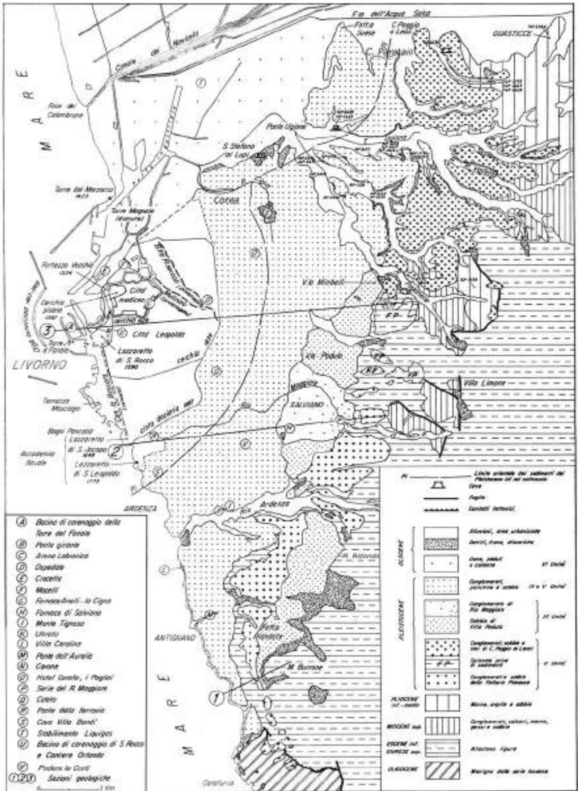
Figura 23 - Carta geologica schematica della Piana di Livorno (da Barsotti et al., 1974).
