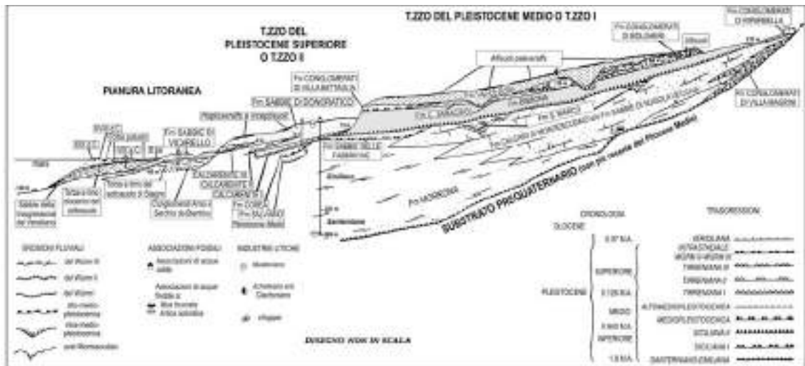
Figura 4 - Schema morfostratigrafico del Pleistocene della Toscana Costiera, ottenuto da tutte le formazioni marine e dalle continentali geograficamente più diffuse (altezze esagerate fortemente rispetto alle lunghezze date non in scala).
