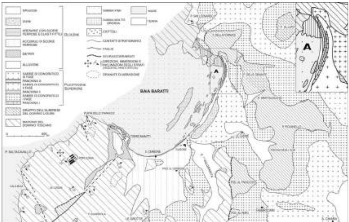
Figura 66 - Carta geologica schematica della Baia Baratti e dintorni (da Cortemiglia et al., 1983).
