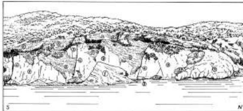
Figura 84 - Parte centrale dell'Isola di Cerboli nel Canale di Piombino. 1 - <Panchina> in primo piano (radicata), 2 - <Panchina> in secondo piano (radicata), 3 - <Panchina> in massi caduti, 4 - Specchi di faglia nel calcare liassico, 5 - <Panchina> appoggiata contro il calcare liassico, 6 - <Panchina> e breccie con croste calcaree di chiusura del ciclo pleistocenico, 7 - Calcare Massiccio (Lias), 8 - Altri elementi della Serie Toscana.
