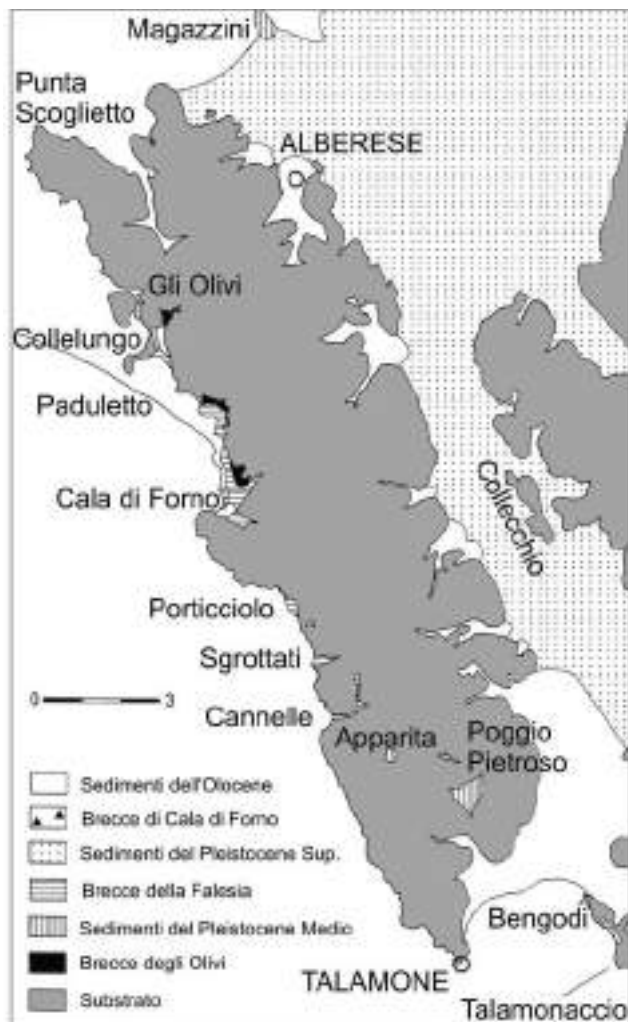
Figura 24 - Carta dei siti del Quaternario nei M. ti dell'Uccellina – Collecchio – Talamonaccio.
