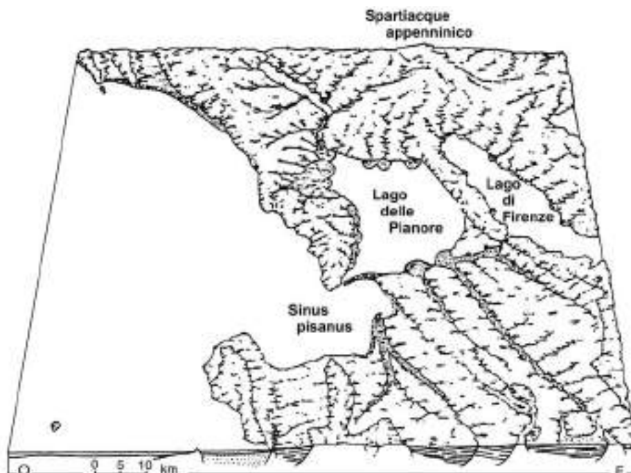
Figura 16 - Stereogramma rappresentativo della paleogeografia dell'area del Valdarno Inferiore nel Pleistocene Inferiore (da Federici e Mazzanti, 1988).
