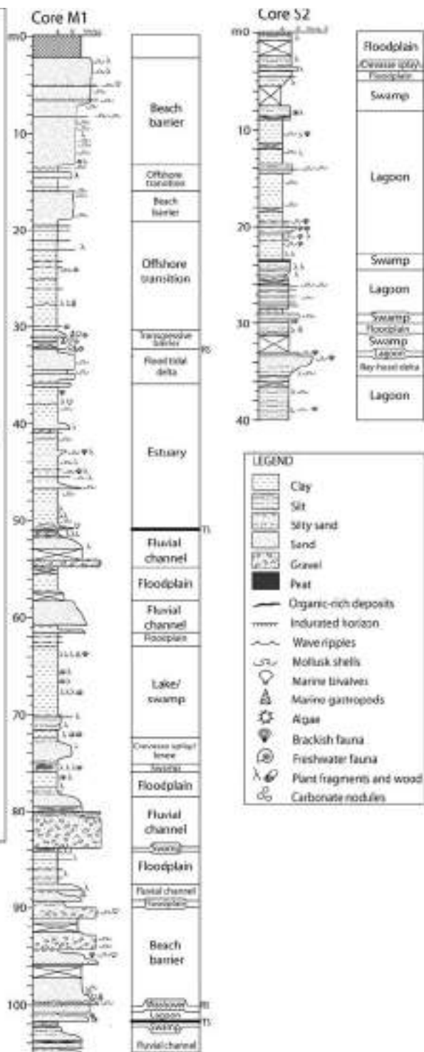
Figura 46 - Stratigrafia e interpretazione delle facies dei Sondaggi M1 e S2 (da Aguzzi et al., 2005).
