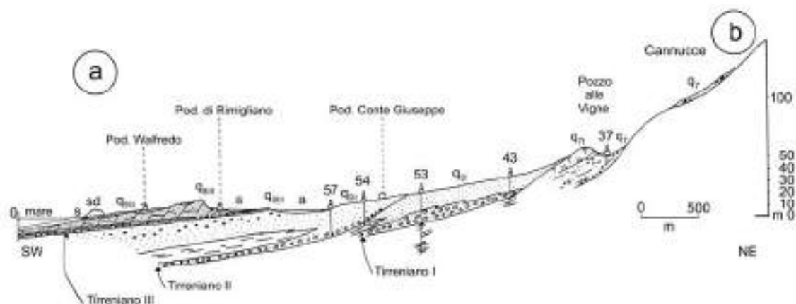
Figura 29 - Sezione geomorfologica localizzata (tra a – b) in Figura 18 per mostrare la stratigrafia del T. ZZO di Palmentello-Lumiere: q 7 - Sabbie di Val di Gori e q 7t - Travertino (Substrato del Pleistocene Medio); q 9I - Sabbie di Donoratico attribuite al Tirreniano I; q 9II - Sabbie di Donoratico attribuite al Tirreniano II; q 8III - Calcareniti e q 9III - Sabbie di Donoratico attribuite al Tirreniano III; sd - Duna e s - Spiaggia (attuali) da Costantini et al. (1995).
