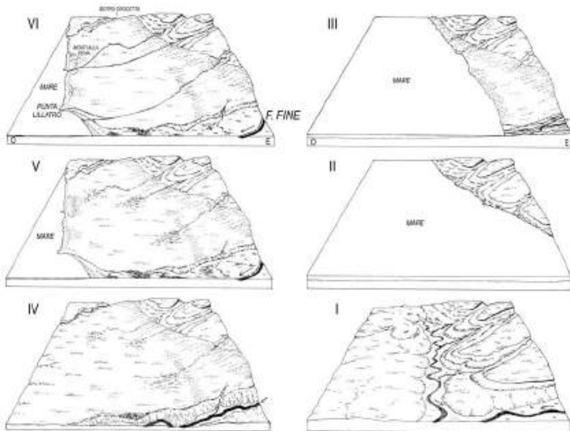
Figura 52 - La Piana di Rosignano Solvay : I - nella situazione precedente alla trasgressione marina del Tirreniano, II - durante il massimo della trasgressione del Tirreniano (OIS 5e), III - durante il massimo della fase (OIS 5c), IV - durante la regressione marina del Würm III, V - durante la trasgressione dell'Olocene prima di ogni intervento umano, VI - nella situazione attuale che mostra la canalizzazione di tutti i corsi d'acqua ma non segna le aree ingombre di edifici abitativi ed industriali che occupano ormai tutta l'area tranne l'estremo lembo meridionale corrispondente all'alveo del F. Fine (da Mazzanti, 1986).
