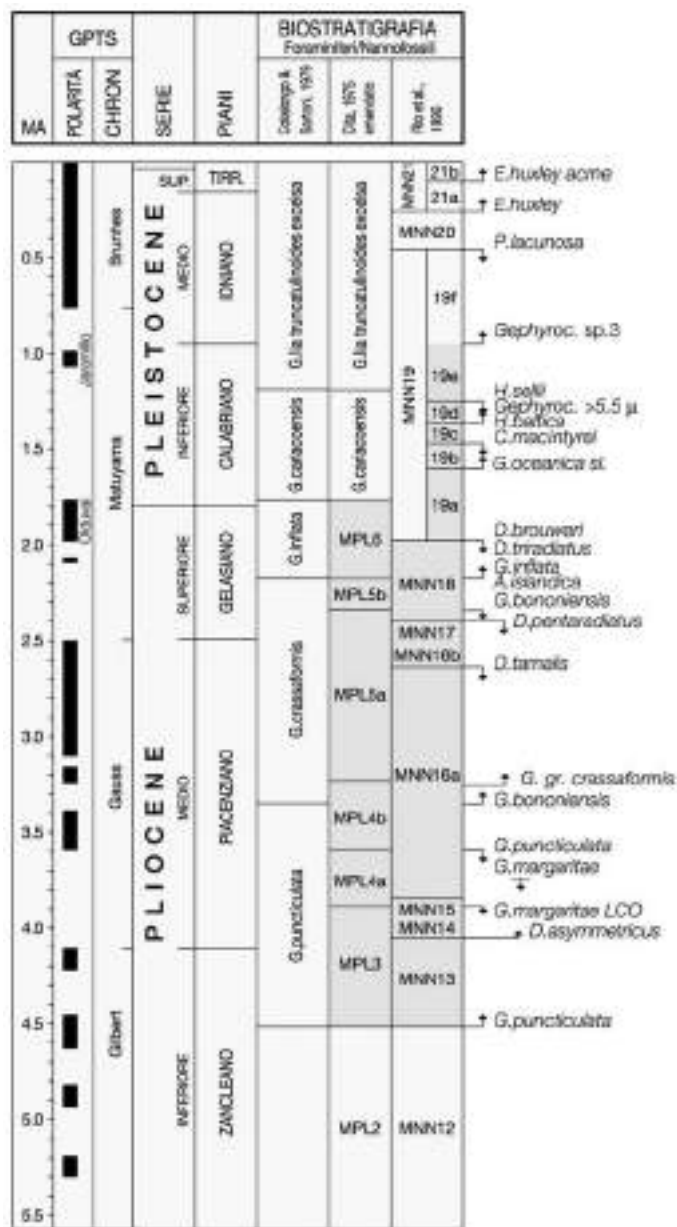
Figura 3 - Successioni cronologiche e biostratigrafiche delle Serie e Piani marini delle Epoche Pliocene e Pleistocene (da Catanzariti et al., 2002).
