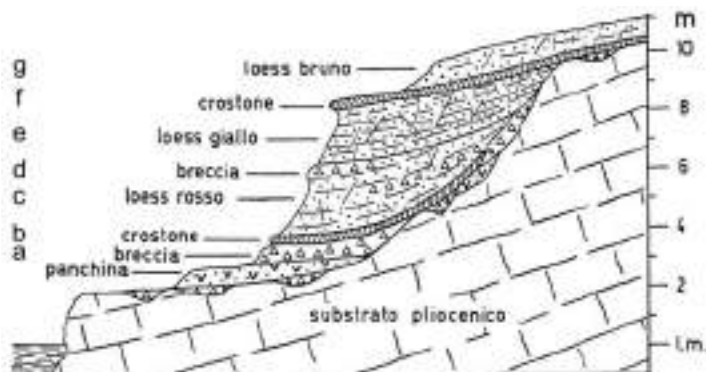
Figura 87 - Schema dei depositi quaternari dell'Isola di Pianosa. a - <Panchina> tirreniana a faune marine; b - Breccia; c - Crostone; d - <Loess rosso> talora con breccie; e - <Loess giallo>; f - Crostone; g - <Loess bruno> (da Colantoni e Borsetti, 1973).
