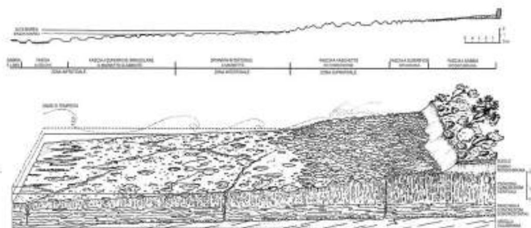
Figura 28 - Stereogramma per mostrare le strutture sedimentarie delle Calcareni di Castiglioncello e le fasce di erosione che si sviluppano sopra la loro superficie superiore per azione, nella fascia supratidale, dell'aerosol marino nei giorni di vento di mare cui si mescolano le acque dolci dei giorni di pioggia e, nelle fasce sommerse, per le azioni della dinamica marina (da Mazzanti e Parea, 1979).
