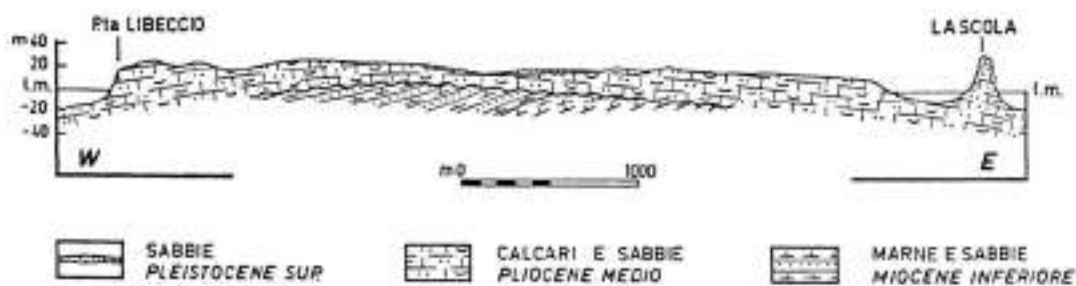
Figura 86 - Carta geologica schematica dell'Isola di Pianosa (da Colantoni e Borsetti, 1973).
