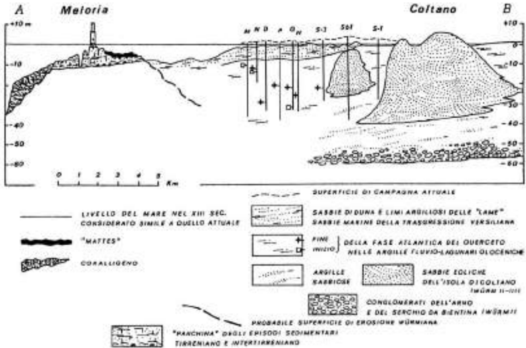
Figura 42 - Sezione geologica tra la Meloria e Coltano. Le altezze sono ingrandite di 100 volte rispetto alle lunghezze per rendere leggibile il disegno (da Mazzanti et al., 1984).
