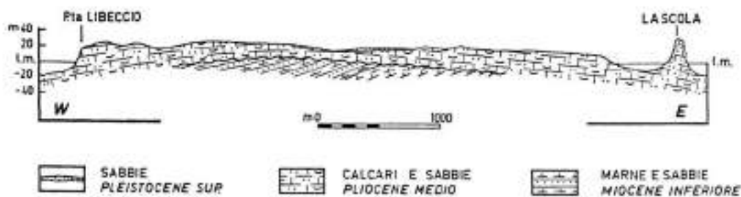
Figura 86 - Carta geologica schematica dell'Isola di Pianosa (da Colantoni e Borsetti, 1973).
