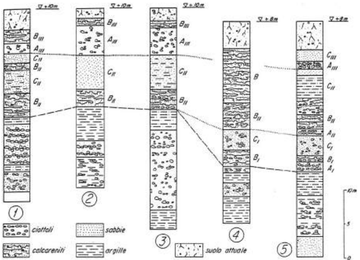
Figura 75 - Sondaggi eseguiti tra S. Vincenzo e La Punticella lungo il retroterra del litorale (Figura 18). La litologia dei vari livelli risulta dall'associazione dei tipi fondamentali mostrati negli appositi riquadri; le lettere A-B-C indicano gli elementi (rispettivamente in prevalenza conglomeratici, calcarenitici e sabbiosi) delle tre sequenze sedimentarie (indicate con i numeri romani a fianco) che si è tentato di rintracciare. La linea a tratti corrisponde con il limite inferiore delle calcareniti e dei ciottoli e conglomerati ad esse associati con significato chiaramente trasgressivo; le linee a puntini indicano i successivi episodi trasgressivi (da Mazzanti et al., 1981).
