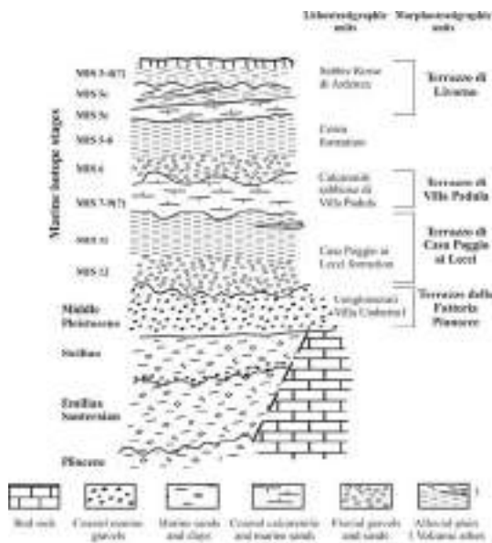
Figura 27 - Stratigrafia del Pleistocene di Livorno secondo Zanchetta et al. (2006).
