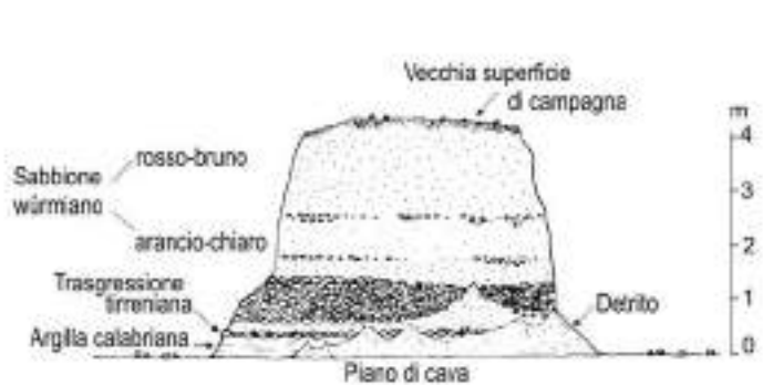
Figura 39 - Residuo della Cava in destra del T. UGIONE , rimasto isolato al centro della Cava per la presenza di un traliccio dell'ENEL.
