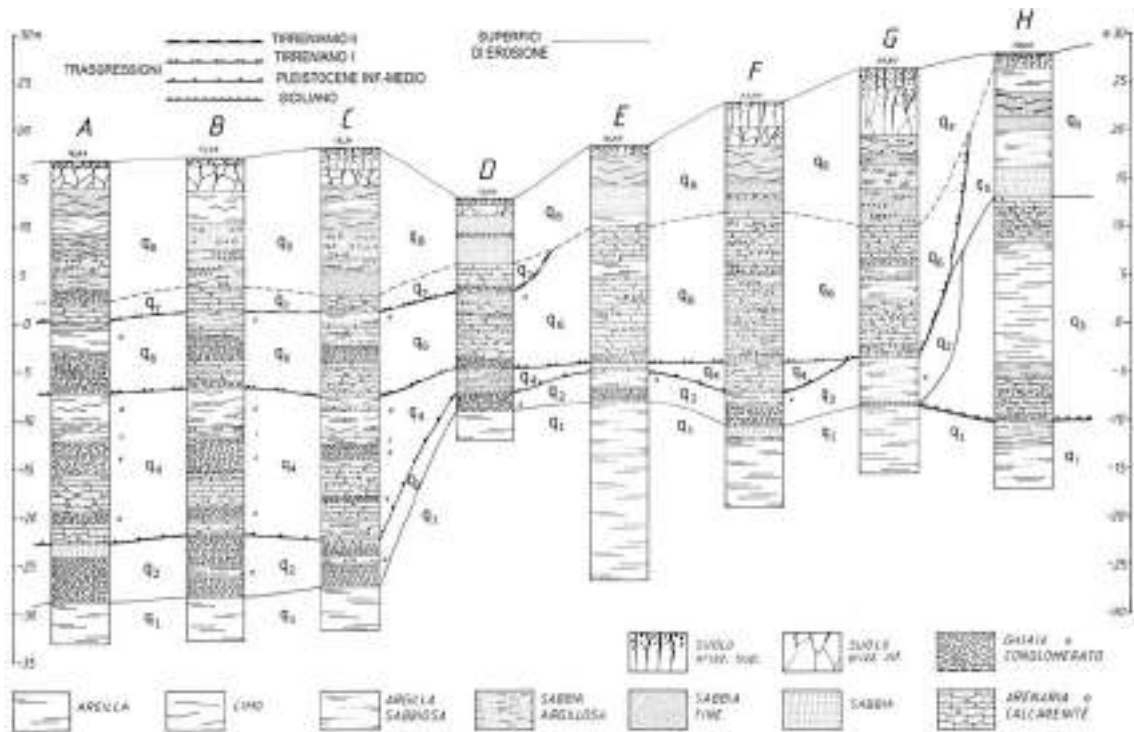
Figura 54 - Stratigrafie dei pozzi dell'interno di Vada; le sigle indicano le seguenti formazioni: q_1 = Fm di Morrone, q_2 = Fm di S. Marco, q_3 = Sabbie delle Fabbriche, q_4 = Fm di C. sa Saracino, q_5 = Sabbie di Val di Gori, q_6 = Calcareniti di Castiglioncello (OIS 5c), q_7 = Calcareniti di Antignano (OIS 5c), q_8 = Sabbie di Donoratico (Würm I e II) (da Bartoletti et al., 1986 con aggiornamento dei nomi e delle sigle formazionali).
