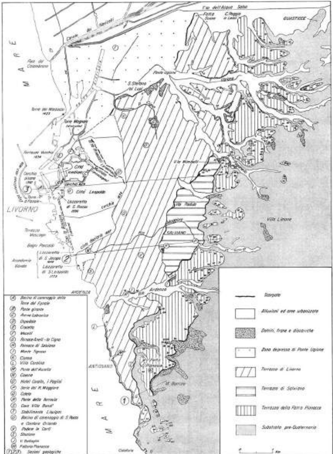
Figura 19 - Carta morfologica schematica della Piana di Livorno (da Barsotti et al., 1974).
