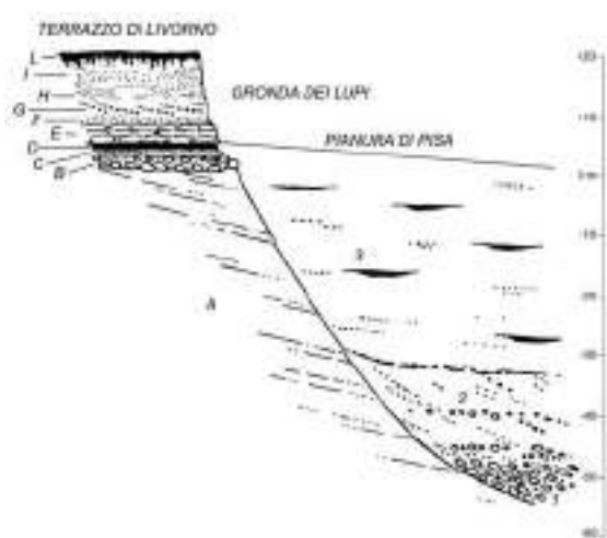
Figura 26 - Successione stratigrafica della <Gronda dei Lupi> (da Fancelli et al., 1986): A - Fm di Morrone; B - Conglomerato; C - Sabbia grigia; D - Argilla continentale di clima freddo; E - <Panchina> con fossili marini; F - Sabbia con fauna salmastra; G - Ghiaino; H - Sabbia grossolana di duna arrossata; I - Sabbia eolica finissima, arrossata, finemente stratificata; L - Suolo contenente industria mustertiana; 1 - Conglomerati dell'Arno e Serchio da Bientina; 2 - Limi fluvio-palustri del sottosuolo; 3 - Limi fluvio-palustri di superficie.
