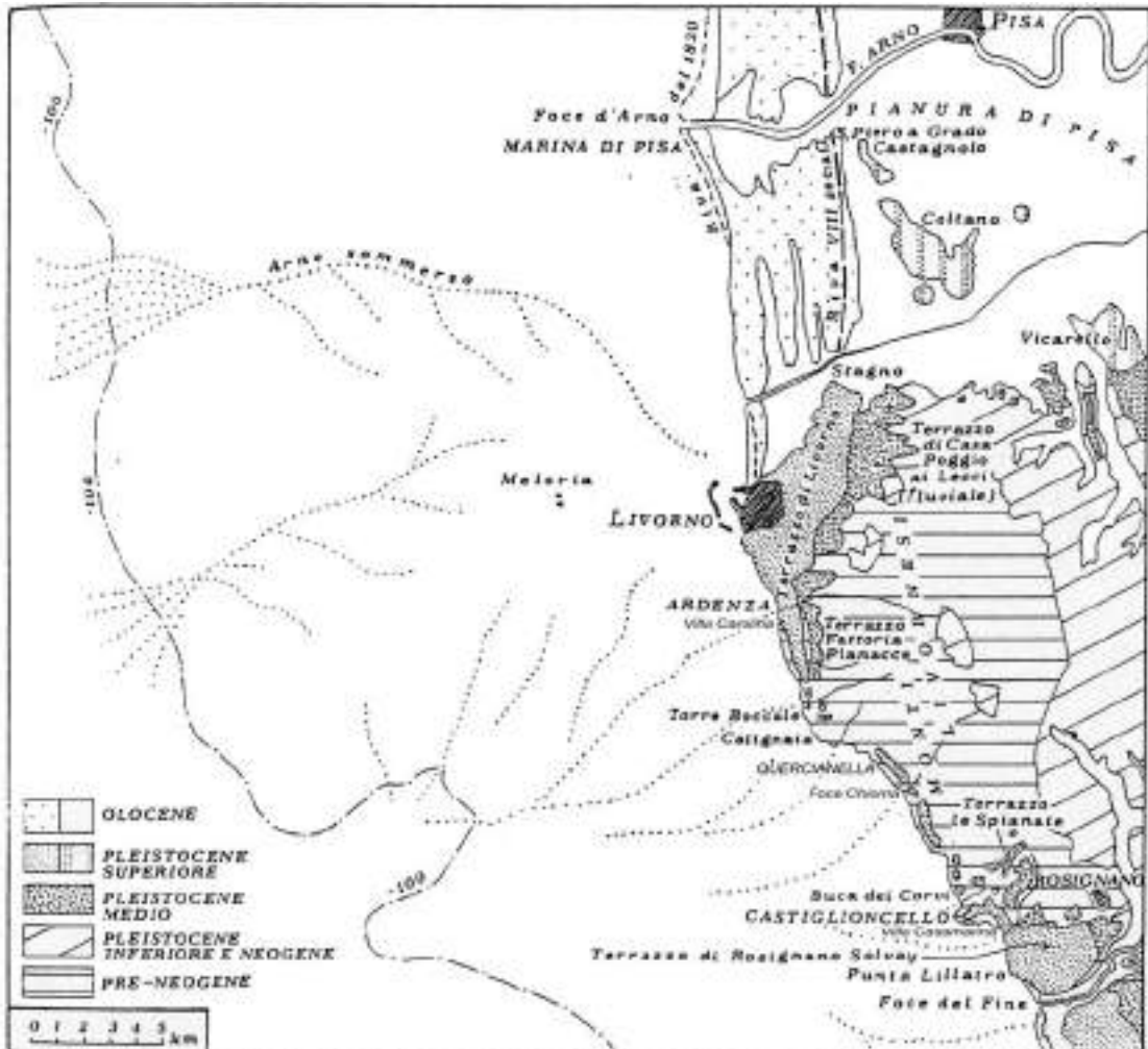
Figura 30 - Carta geomorfologica schematica del litorale compreso tra le foci dei fiumi Arno e Fine (da Galoppini et al., 1996).
