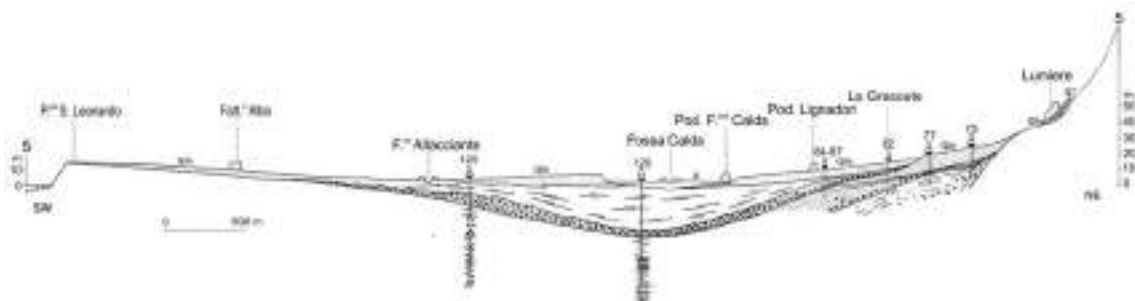
Figura 64 - Sezione geologica tra il P. gio S. Leonardo e Lumiere per mostrare la possibilità di rintracciare tre cunei sedimentari del Pleistocene Superiore (da Costantini et al., 1995).
