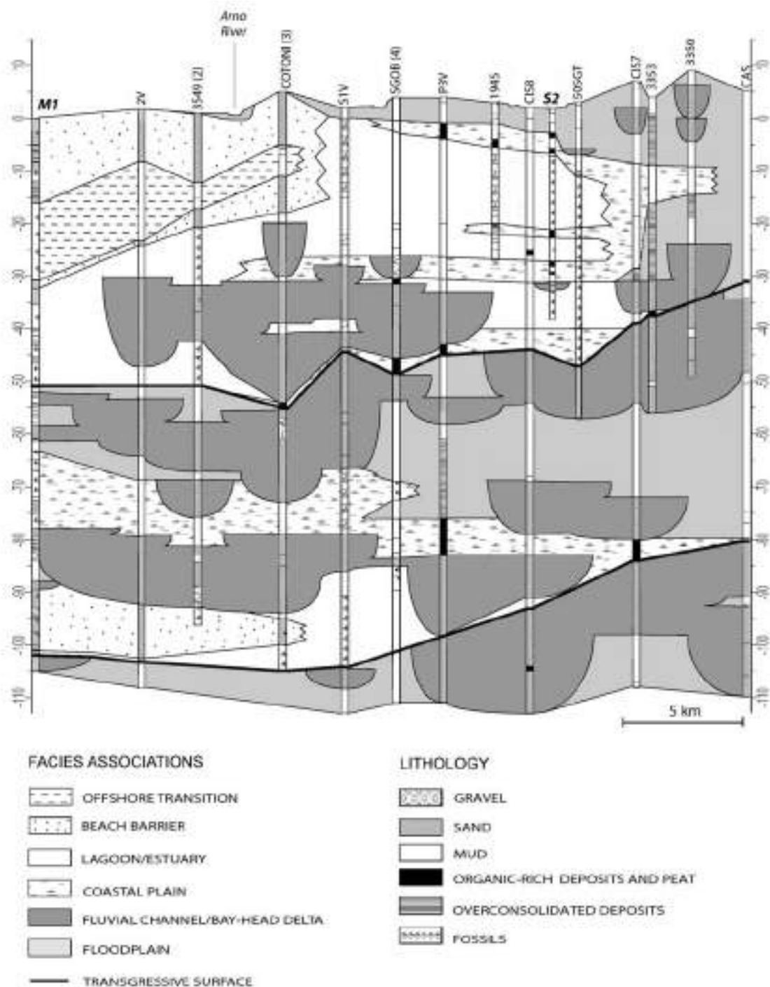
Figura 48 - Stratigrafia del sottosuolo della Pianura del Valdarno inferiore (secondo Aguzzi et al. 2005).
