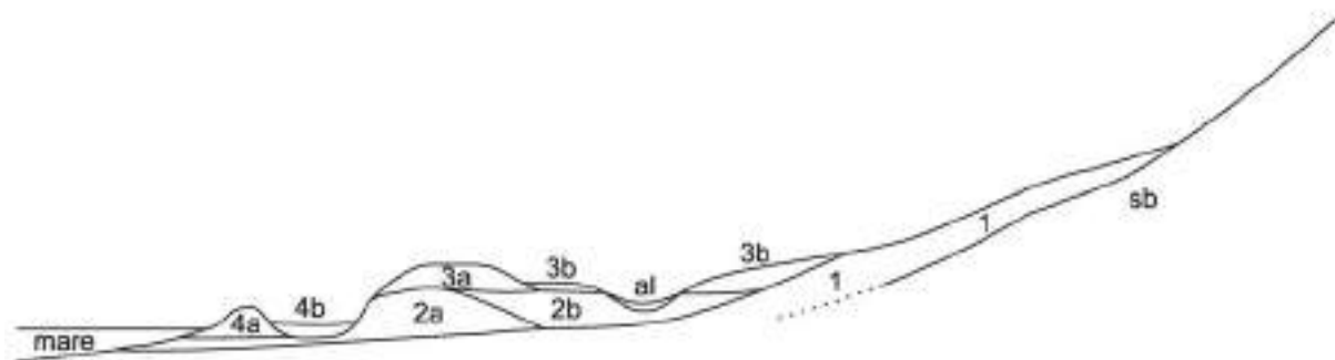
Figura 81 - Sezione geologica attraverso il Lago di Burano; sb – Substrato pre-pleistocenico; 1 – Conglomerati e sabbie alluvionali (Pleistocene Medio e/o Superiore?); 2a - Sabbie e conglomerati marini, 2b – Sabbie fini siltose e limi marini (Pleistocene Superiore – 125 ka); 3a - Sabbie a stratificazione incrociata, 3b – Sabbie sottilmente calcaree e ricche di vulcaniti (Pleistocene Superiore – 110 ka); 4a – Sabbie eoliche, 4b – Sedimenti lacustri (Olocene); al – Sedimenti alluvionali (da Aldinucci et al., 2004).
