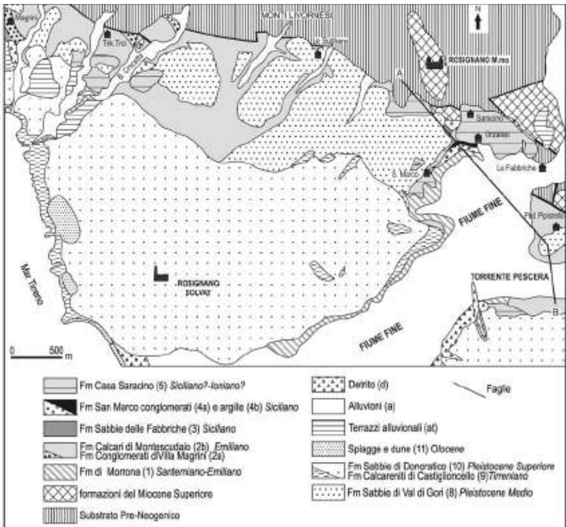
Figura 11 - Carta geologica schematica dell'area centrale del Comune di Rosignano M. mo (da Dall'Antonia et al., 2005).
