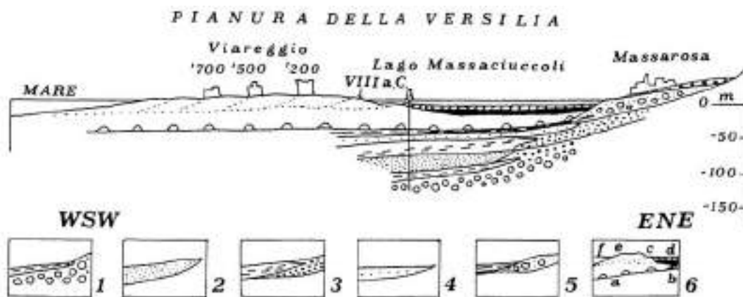
Figura 43 - Sezione geologica (non in scala) fra Viareggio e Massarosa, ricostruita sulla base dei dati di numerosi sondaggi (Federici, 1993), privi di datazioni radiometriche per le parti sottostanti ai depositi del Würm III: 1 - Depositi attribuiti al Würm I (non raggiunti dal sondaggio ENEA), 2 - Depositi attribuiti all'interstadio Würm I-II ma risultati dell'OIS 5e dalle datazioni ENEA (Antonioli et al., 2000); 3 - Depositi attribuiti al Würm II di facies continentale di datazione incerta dopo i risultati del sondaggio ENEA; 4 - Depositi attribuiti all'interstadio Würm II-III e 5 - Depositi attribuiti al Würm III rimangono entrambi, dopo le determinazioni di età radiometriche ENEA, nell'approssimazione di un'età convenzionale >53500 anni B.P. fino al campione (ancora sondaggio ENEA) proveniente da -34,0 m e con età calibrata di 9590 \pm 60 anni B.P. in argilla limosa continentale, quindi già rientrante nell'Olocene; 6 - trasgressione del Versiliano, nel sondaggio ENEA inizia a -30 m col campione datato 8419 \pm 48 (Menozzi et al., 2002); questa trasgressione si è spinta fino al cono di deiezione sul quale è costruita Massarosa ma già nell'VIII sec. a.C. era emerso il lido che separava dal mare il Lago di Massaciuccoli; infine le torri della Guardia costiera di Viareggio, costruite man mano che la spiaggia progradava, marcano la posizione di quest'ultima nel 1200, nel 1500 e nel 1700 (da Mazzanti, 1994).
