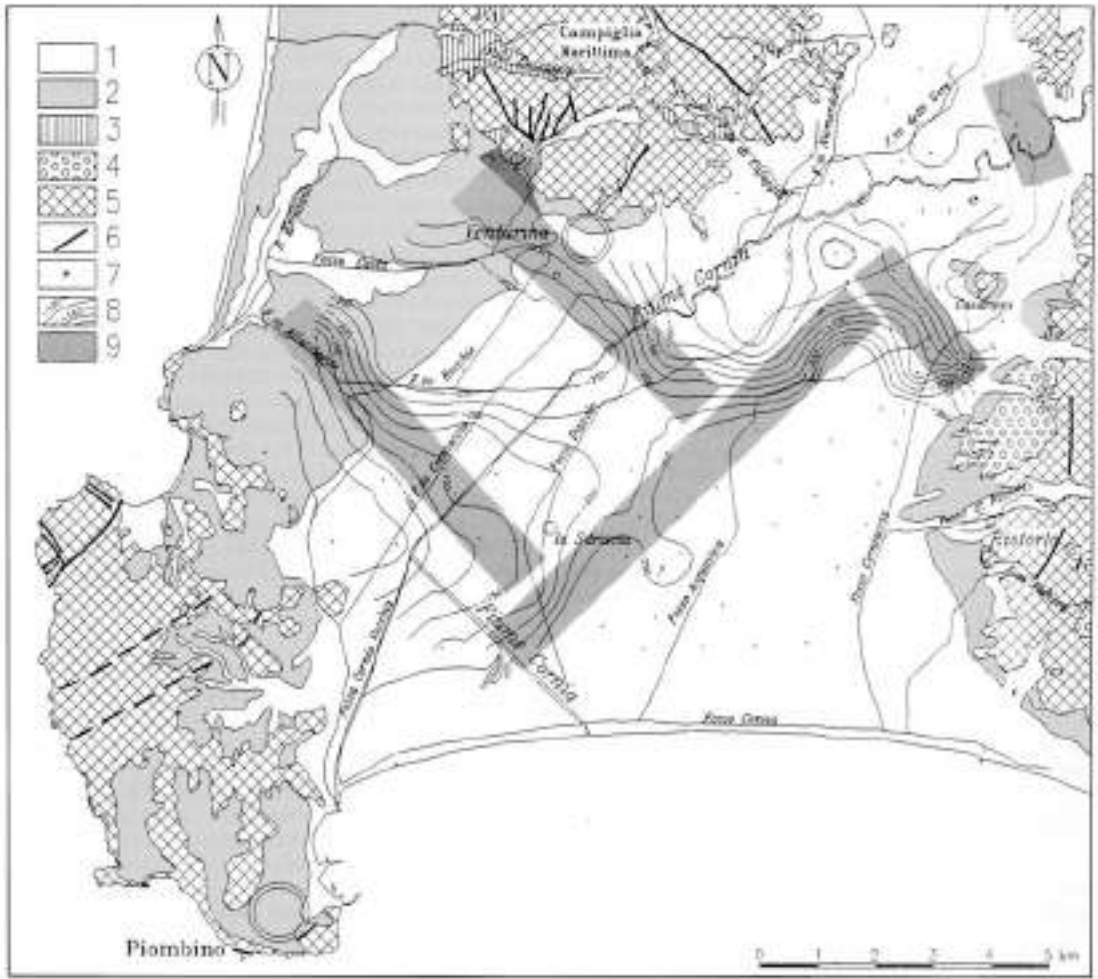
Figura 61 - Carta delle isoipse delle formazioni anteriori al Miocene Superiore (Superficie sepolta Se_1 . 1 - 7 come in Figura 60; 8 - isoipse del tetto delle formazioni anteriori al Miocene Superiore; tratti a notevole ripidità della Superficie Se_1 (verosimilmente corrispondenti a faglie o fasci di faglie).
