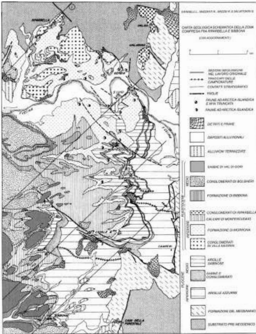
Figura 10 - Carta geologica schematica della zona compresa fra Riparbella e Bibbona (da Giannelli et al., 1981b, con aggiunte e lievi modifiche).
