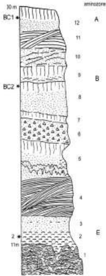
Figura 49 - Stratigrafia della sezione della Buca dei Corvi; 1 – Ofioliti del substrato pre-Quaternario, 2 – deposito fossilifero marino, 3 – suolo rosso, 4 – eolianite, 5 – suolo bruno, 6 – colluvium, 7 – suolo, 8 – sabbie rosicce, 9 – eolianite rossa alterata, 10 – colluvium eolico, 11 – sabbie eoliche “massive” (termine in netto contrasto con quanto segnato in figura!) (da Hearty e Dai Pra, 1986).
