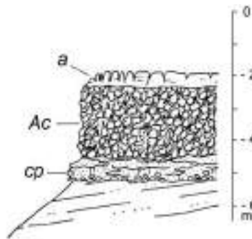
Figura 38 - Particolare della Sezione B di Figura 33, il significato delle lettere è nel testo.
