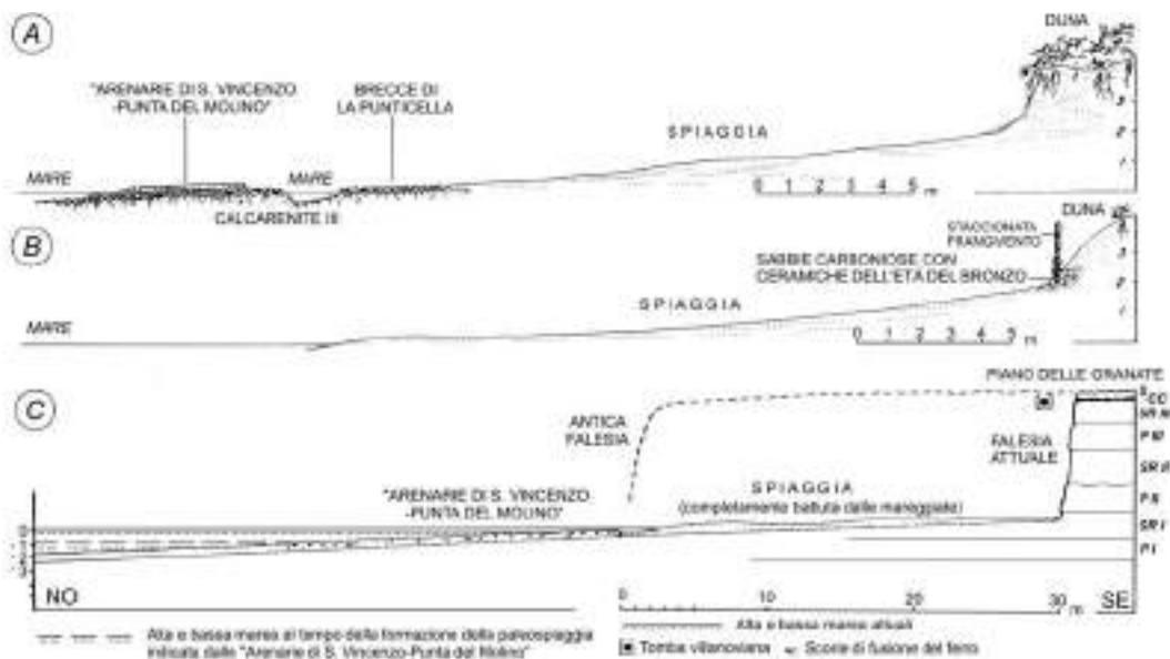
Figura 59 - A – Sezione geologica in corrispondenza de La Punticella a Sud di S. Vincenzo per mostrare i rapporti tra Breccie di La Punticella ed Arenarie di S. Vincenzo-Punta Molino. Entrambe queste formazioni contengono abbondanti clasti della fusione dei materiali ferrosi elbani (da Mazzanti et al., 1981). B – Sezione posta circa 75 m a Sud de La Punticella, in corrispondenza del piccolo affioramento di sabbie brune, leggermente carboniose e con frammenti ceramici dell'Età del Bronzo (da Fedeli e Galiberti, 1979). C – Sezione attraverso il litorale della Baia Baratti all'altezza del Piano delle Granate; P I – <panchina> I; SR I – sabbie rosse I; P II – <panchina> II; SR II – sabbie rosse II; P III <panchina III>; SR III – sabbie rosse III; CC – ceneri e carboni; S – suolo (da Pasquinucci e Mazzanti, 1987).
