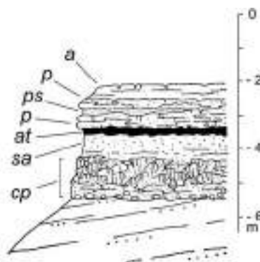
Figura 36 - Particolare della Sezione E di Figura 33. il significato delle lettere è nel testo.
