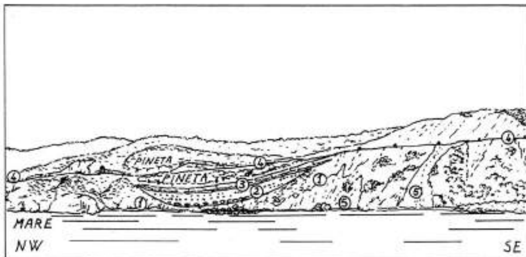
Figura 65 - Visione panoramica della sezione del Pleistocene Superiore de I Tufi sulla costa occidentale del P. torio di Piombino: 1 – Arenaria Macigno del substrato; 2 – Banco di base del Pleistocene Superiore formato da grandi ciottoli di Macigno in basso e da sabbia grossolana a matrice argillosa con livelli di breccie stratificate; 3 – Banco superiore di <Panchina> di facies marina in basso ed eolica in alto; 4 – Profilo della strada – sentiero; 5 – Materiali franati.
