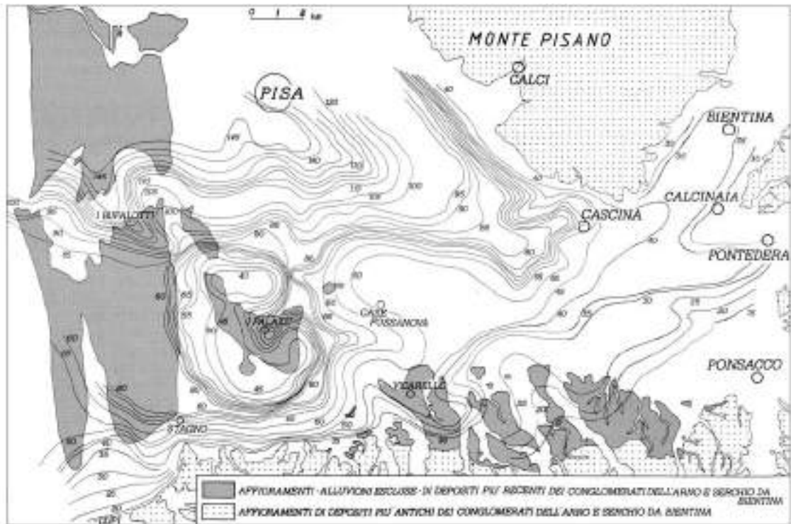
Figura 47 - Posizione del livello dei Conglomerati dell'Arno e Serchio da Bientina nel sottosuolo della Pianura Pisana (da Fancelli et al. 1986).
