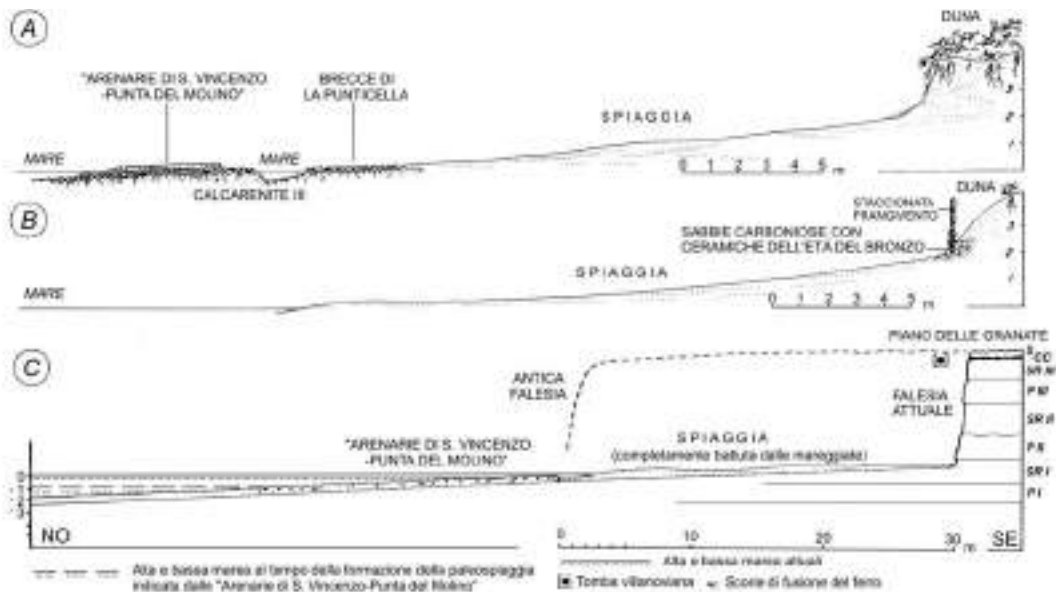
Figura 59 - A – Sezione geologica in corrispondenza de La Punticella a Sud di S. Vincenzo per mostrare i rapporti tra Breccie di La Punticella ed Arenarie di S. Vincenzo-Punta Molino. Entrambe queste formazioni contengono abbondanti clasti della fusione dei materiali ferrosi elbani (da Mazzanti et al., 1981). B – Sezione posta circa 75 m a Sud de La Punticella, in corrispondenza del piccolo affioramento di sabbie brune, leggermente carboniose e con frammenti ceramici dell'Età del Bronzo (da Fedeli e Galiberti, 1979). C – Sezione attraverso il litorale della Baia Baratti all'altezza del Piano delle Granate; P I – <panchina> I; SR I – sabbie rosse I; P II – <panchina> II; SR II – sabbie rosse II; P III <panchina III>; SR III – sabbie rosse III; CC – ceneri e carboni; S – suolo (da Pasquinucci e Mazzanti, 1987).
