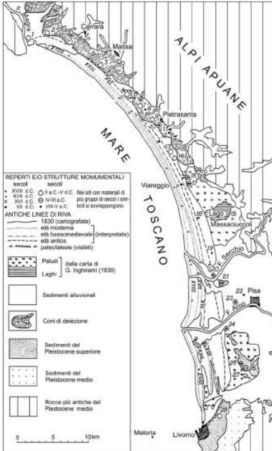
Figura 44 - Lineamenti geomorfologici essenziali della Versilia, in relazione alla posizione dei siti archeologici più significativi per il tracciamento delle antiche linee di riva. 1 – Bocca di Magra, 2 – Luni, 3 – Avenza, 4 – Lago di Porta, 5 – Centoquindici, 6 – Cafaggio, 7 – Frasso, 8 – Pozzi-Querceta, 9 – Ponterosso e Crocialetto, 10 – Pisanica, 11 – Baccatoio, 12 – Traversagna, 13 – Bucine, 14 – Ortacci, 15 – Migliarina, 16 – Cava S.A.P.I.L., 17 – Cava S.I.S.A., 18 – Torre del Lago, 19 – Troncolo, 20 – Isola di Migliarino (Cava Mori), 21 – Palazzetto, 22 – Area Scheibler, 23 – Barbaricina, 24 – S. Piero a Grado, 25 e 26 – Coltano, 27 – Stagno, 28 – S. Stefano ai Lupi (da Mazzanti et al., 1990).
