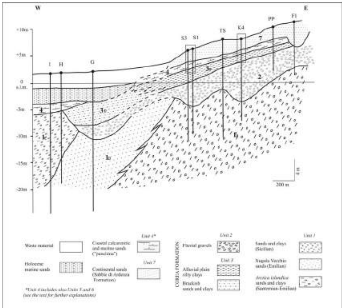
Figura 25 - Stratigrafie dei sondaggi studiati lungo il bordo NO del Terrazzo di Livorno (da Zanchetta et al., 2006).
