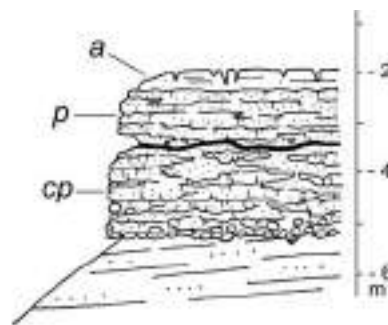
Figura 35 - Particolare della Sezione A di Figura 33, il significato delle lettere è nel testo.
