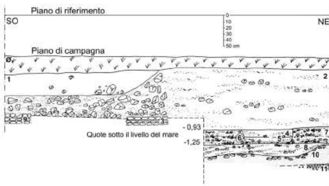
Figura 57 - Sezione lungo il saggio stratigrafico di S. Gaetano di Vada: \emptyset – terreno agricolo; 1 – strato di manipolazione antropica recente; 2 – sabbia mista a malta disfatta, ciottoli di <Panchina> e materiale eterogeneo anche moderno; 3 – fondazione del muro perimetrale orientale degli horrea ; 4 – sabbia a granuli fini mista a rari piccoli ciottoli appiattiti, di spiaggia, e a scarsi frammenti in ceramica d'impasto; 5 – sedimento analogo al precedente, ancora documentante la frequentazione antropica; 6 – fossa grosso modo circolare; 7 – sabbia con piccoli ciottoli di forma irregolare, mista a numerosissimi fossili di ambiente lagunare a comunicazione con il mare aperto; 8 – sabbia a granuli di dimensioni medie con alcuni fossili (analoghi ai precedenti), lenti arrossate, carboncini e frammenti di ceramica d'impasto; 9 – parte inferiore di un muro divisorio interno degli horrea ; 10 – sabbia a granuli fini misti a numerosissimi frammenti di ceramica d'impasto; 11 – ghiaia a piccoli ciottoli irregolari che corrisponde con il livello della falda freatica (da Mazzanti et al., 1995).
