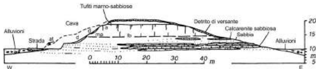
Figura 17 - Sezione della cava presso la Badia di Collesalveti. Le calcareniti sabbiose con fossili marini intercalate alle sabbie di base nella cava appartengono alle Sabbie di Nugola Vecchia; la superficie lb di base del banco marno-argilloso ( ma ) è coperta da un sottile manto di detrito ( d ). La parte alta di questo banco termina con delle argille grigio-perla ( a ) che contengono già vetro vulcanico. Quest'ultimo è abbondante nel banco di cineriti marno-sabbiose al tetto della successione litologica (da Lazzarotto et al., 1990).
