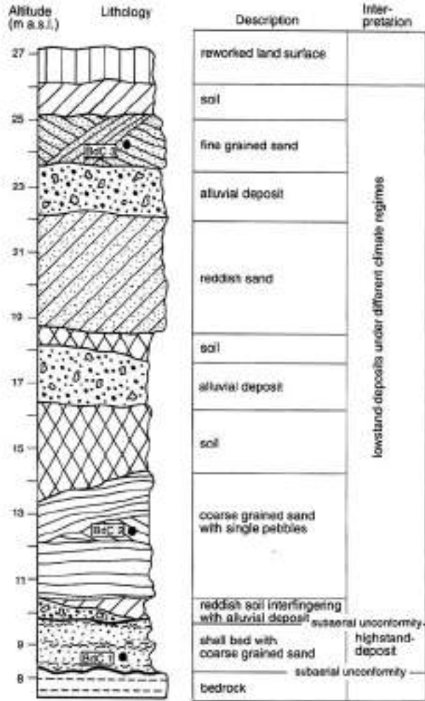
Figura 50 - La sezione della Buca dei Corvi, secondo Barbara Mauz (1999).
